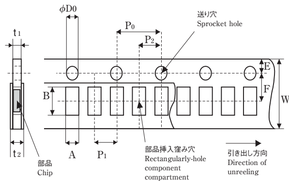
角穴パンチキャリアテープ Rectangularly Punching Carrier Tape (2mm pitch)
